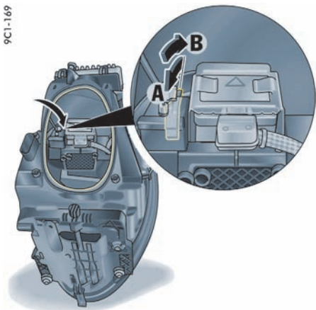
右侧大灯
