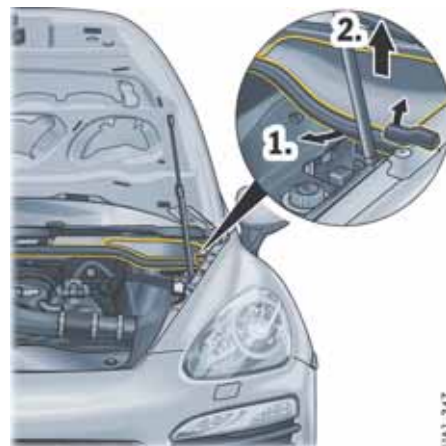
打开发动机舱内的保险丝盒盖
