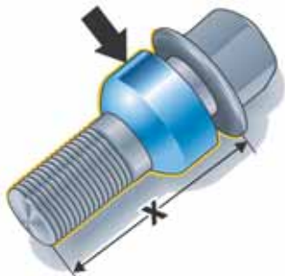
带蓝色球面盖环的长螺栓
